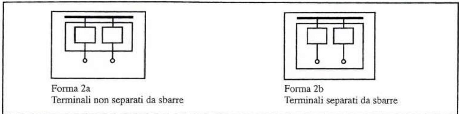
Forma 2: segregazione delle sbarre dalle unità funzionali
