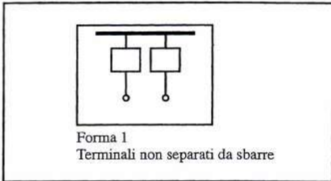
Forma 1: nessuna segregazione interna
