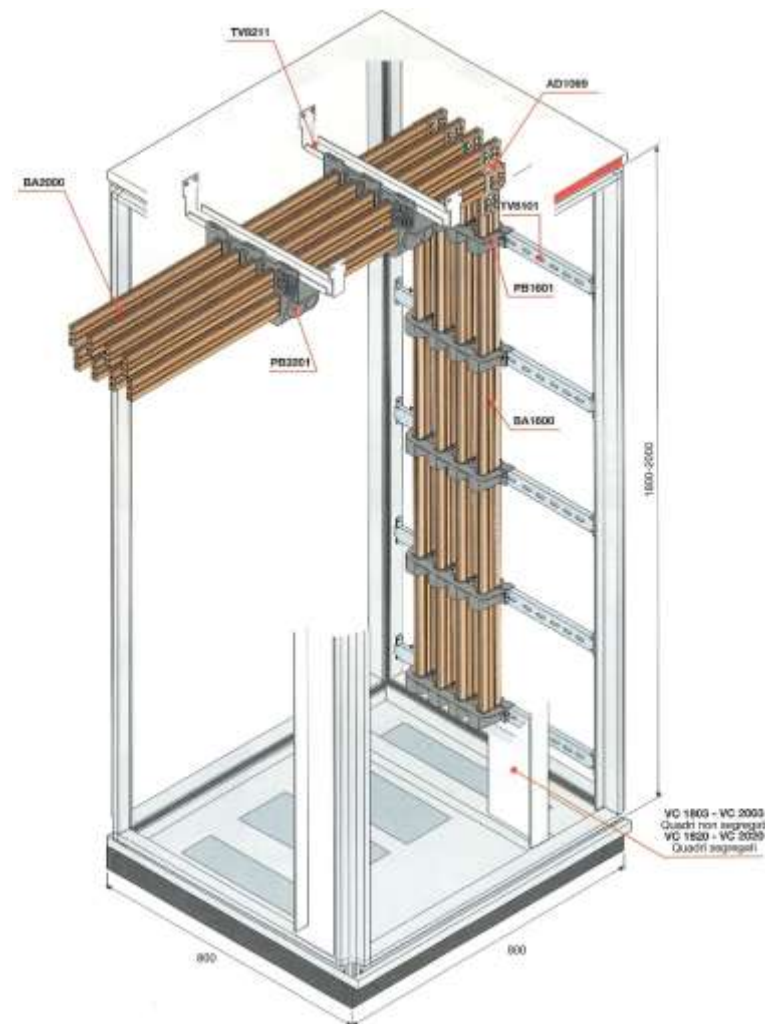
Esempio di sbarre (o barre) sagomate
